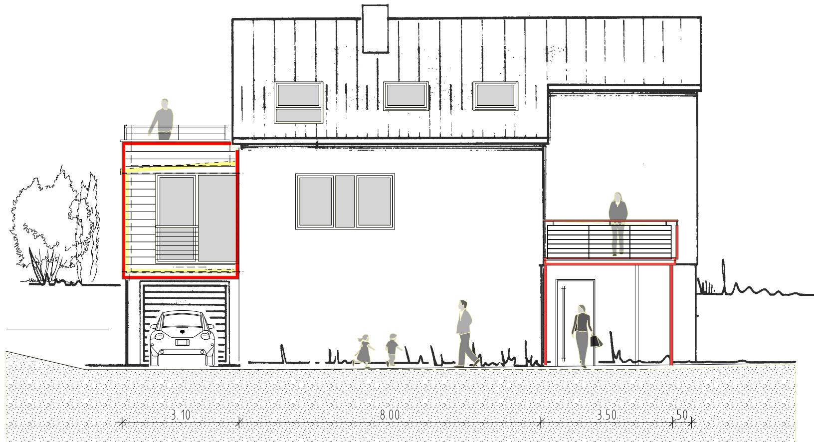
Ansicht West
